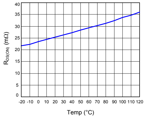
LNFET R_{\text{DS(ON)}} vs. Temp
