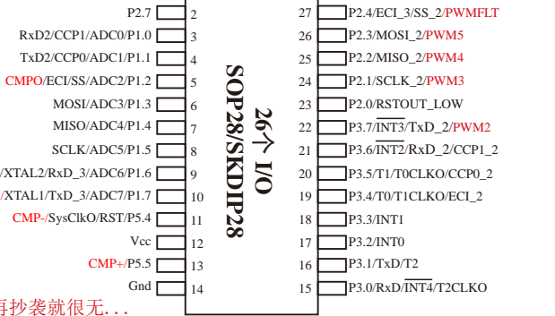
SOP28/SKDP28
