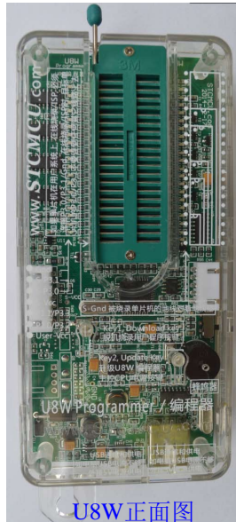
U8W正面图
