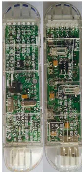
U8-Mini正面图
