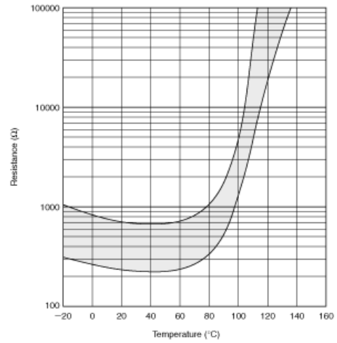
电阻-温度特性范围(参考)
