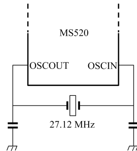
图 10. 石英晶体的连接
