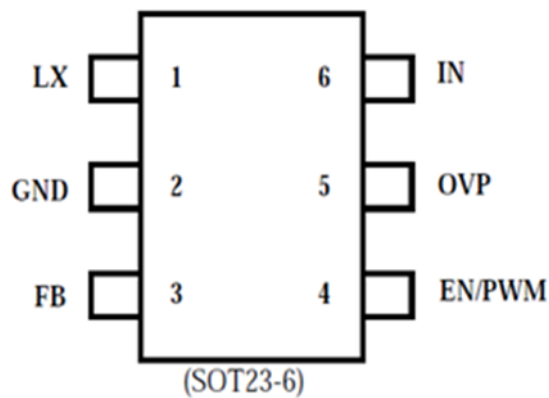
SOT23-6
