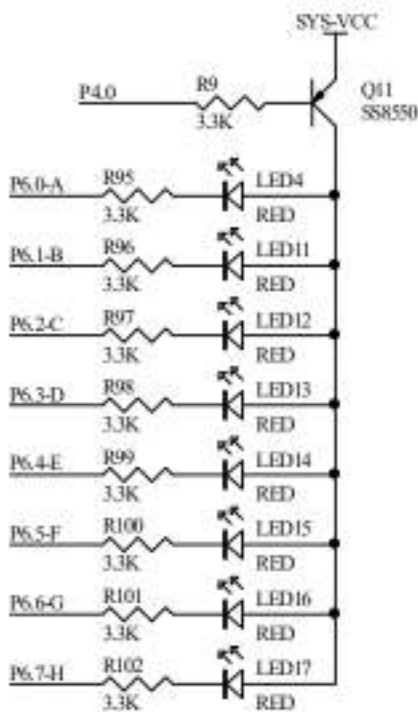
8 个独立 LED 指示灯实验
