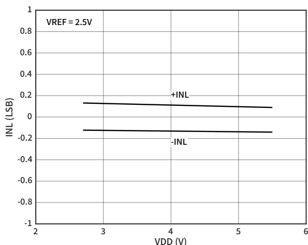
图 3 INL 误差与 VDD 的关系
