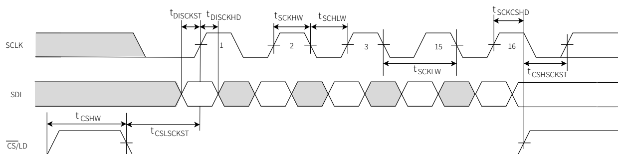
图 1 SPI 时序图
