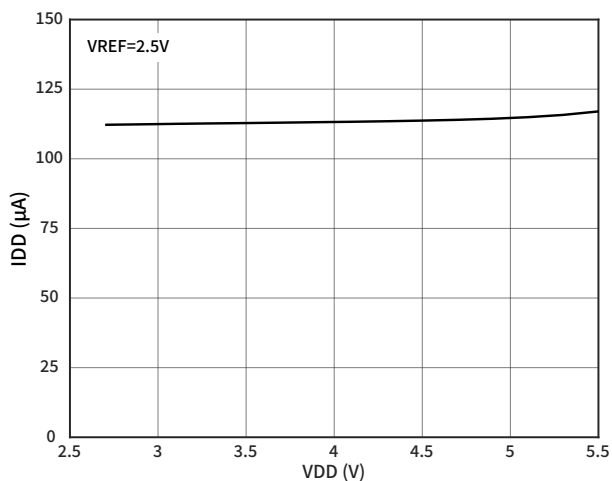
图 14 IDD 与 VDD 的关系
