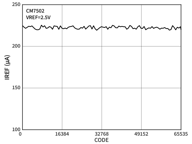
图 9 IREF 与 CODE (CM7502) 的关系
