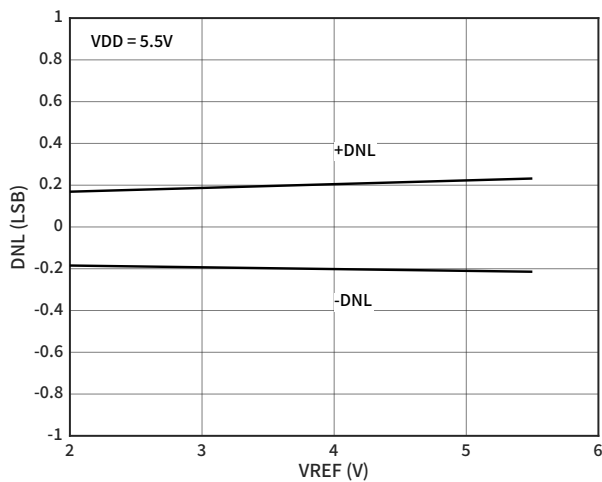
图 7 DNL 误差与 VREF 的关系
