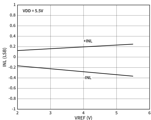
图 4 INL 误差与 VREF 的关系
