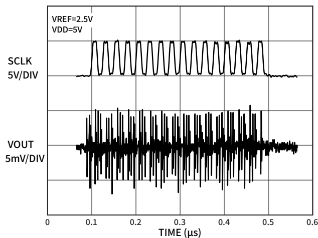
图 17 数字馈通
