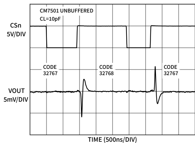
图 18 主进位翻转毛刺脉冲 (CM7501)
