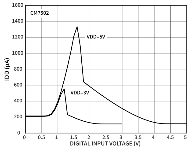
图 13 IDD 与 VIH 的关系 (CM7502)
