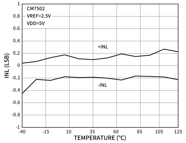
图 21 INL 误差的温度特性 (CM7502)
