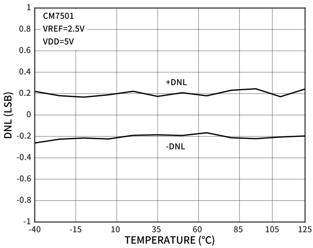
图 22 DNL 误差的温度特性 (CM7501)
