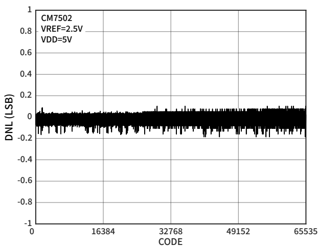
图 5 DNL 误差 (CM7502)
