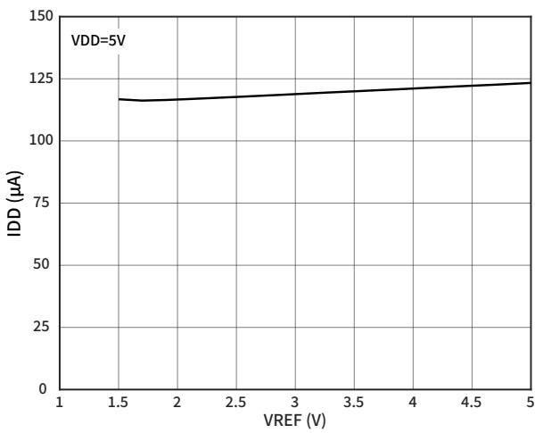
图 10 IDD 与 VREF 的关系 (VDD = 5V)
