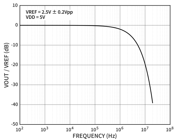
图 16 VOUT/VREF 与频率的关系
