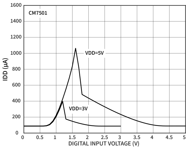
图 12 IDD 与 VIH 的关系 (CM7501)
