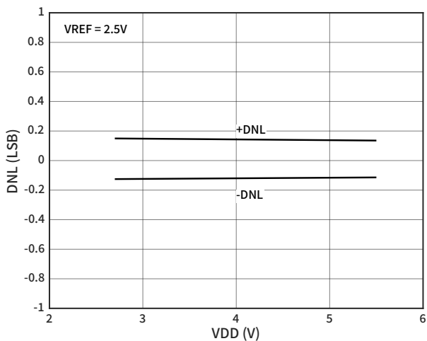
图 6 DNL 误差与 VDD 的关系
