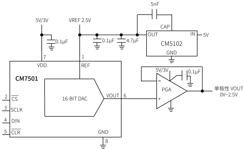
图 27 典型连接 (CM7501)
