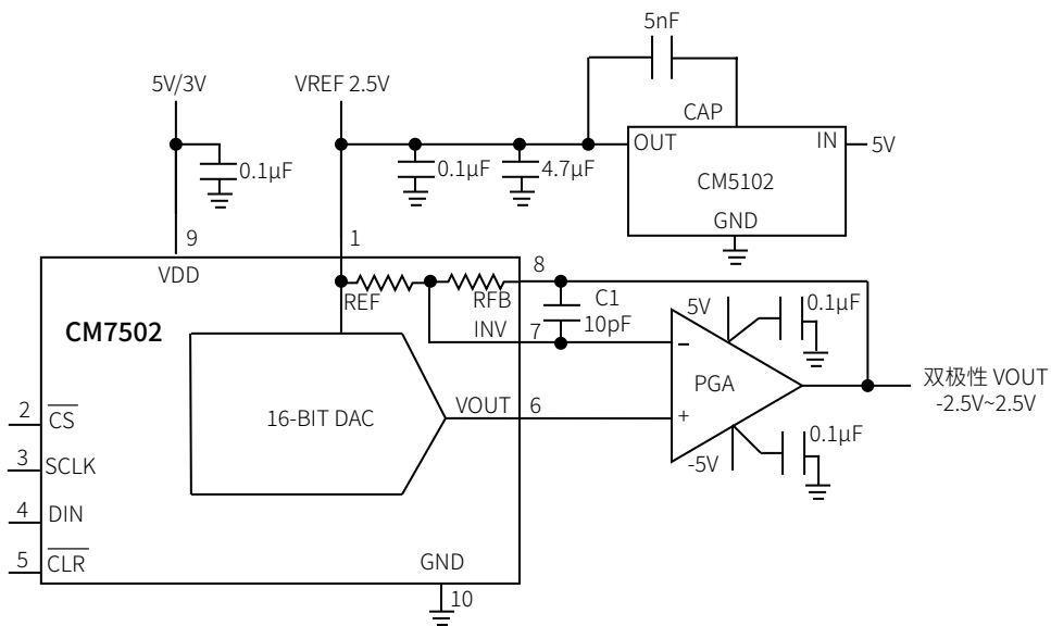
图 26 典型连接 (CM7502)
