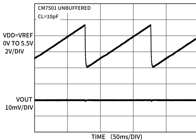
图 15 VOUT 与 VDD = 0V 到 5.5V (上电复位功能, CM7501)
