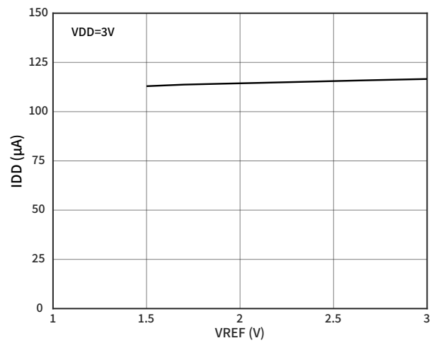
图 11 IDD 与 VREF 的关系 (VDD = 3V)
