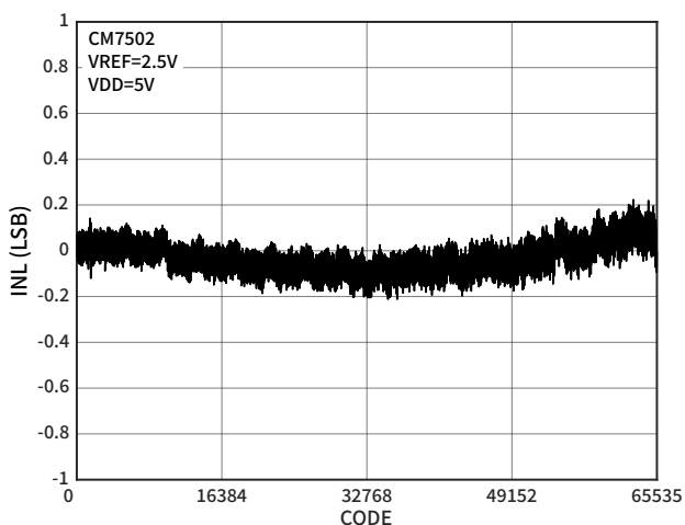
图 2 INL 误差 (CM7502)
