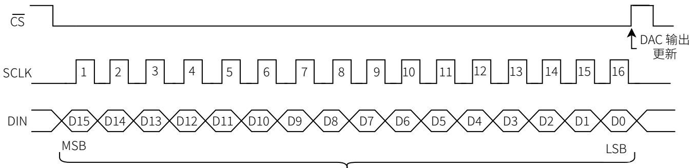
图 25 时序图
