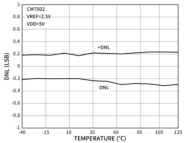
图 23 DNL 误差的温度特性 (CM7502)
