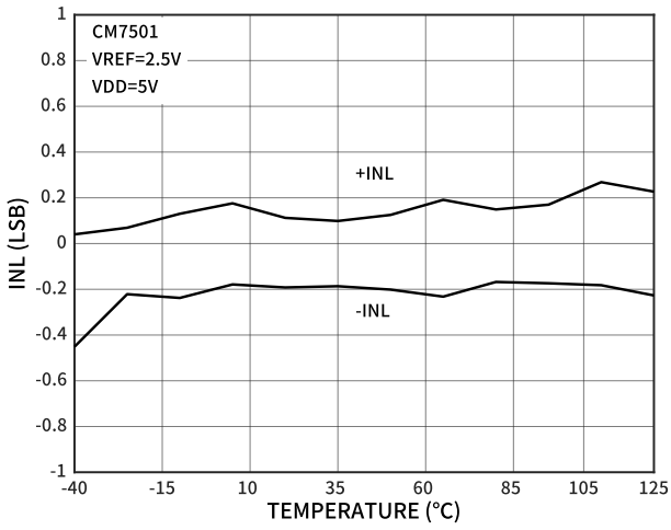
图 20 INL 误差的温度特性 (CM7501)
