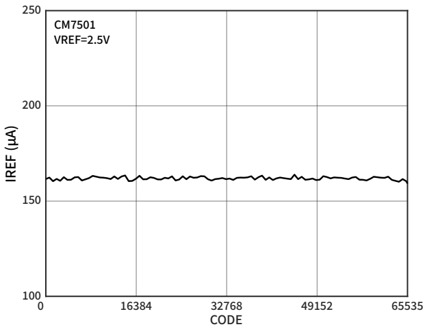
图 8 IREF 与 CODE (CM7501) 的关系
