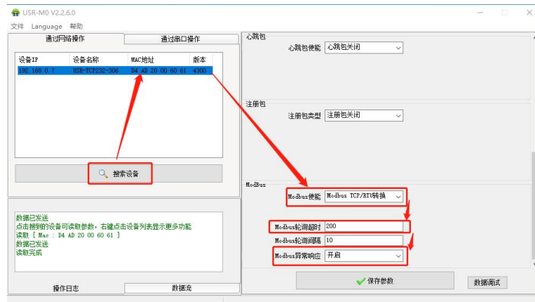
图 21. 软件设置 Modbus 协议转换
