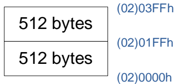
SC92F759X EEPROM Sector 分区示意
