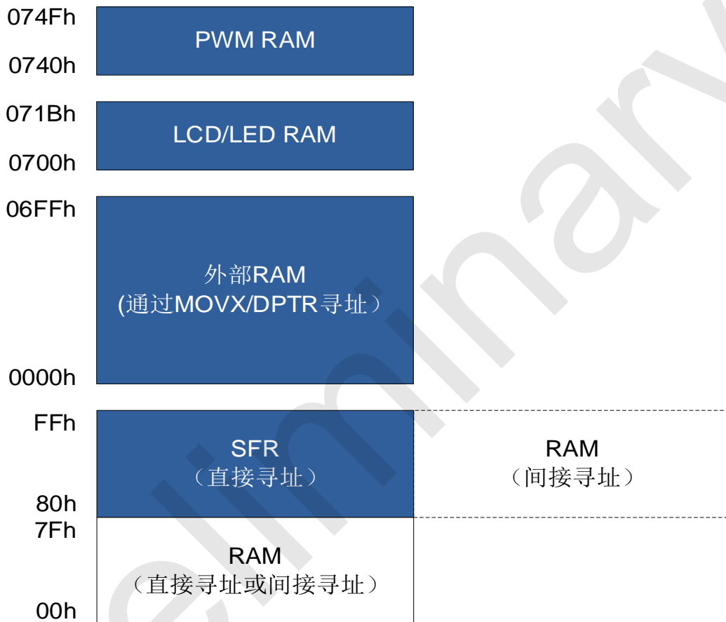
SRAM 结构图
