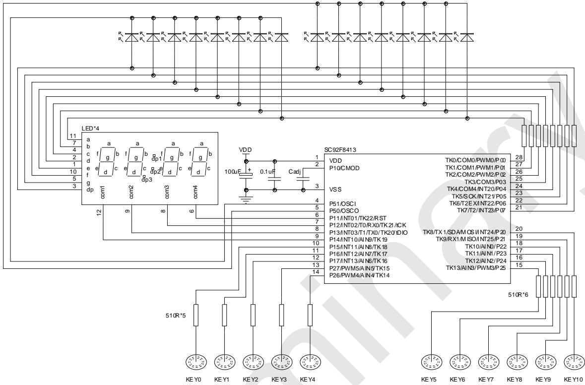
SC92F8413 Touch Key 应用电路图
