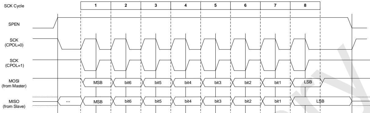
CPHA = 1 数据传输图
