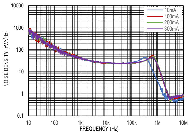
图 19. 输出噪声谱密度, V_{IN}=5\text{V} , V_{OUT}=3.3\text{V}
