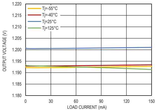
图 10. 1.2V 输出电压和负载电流的关系
