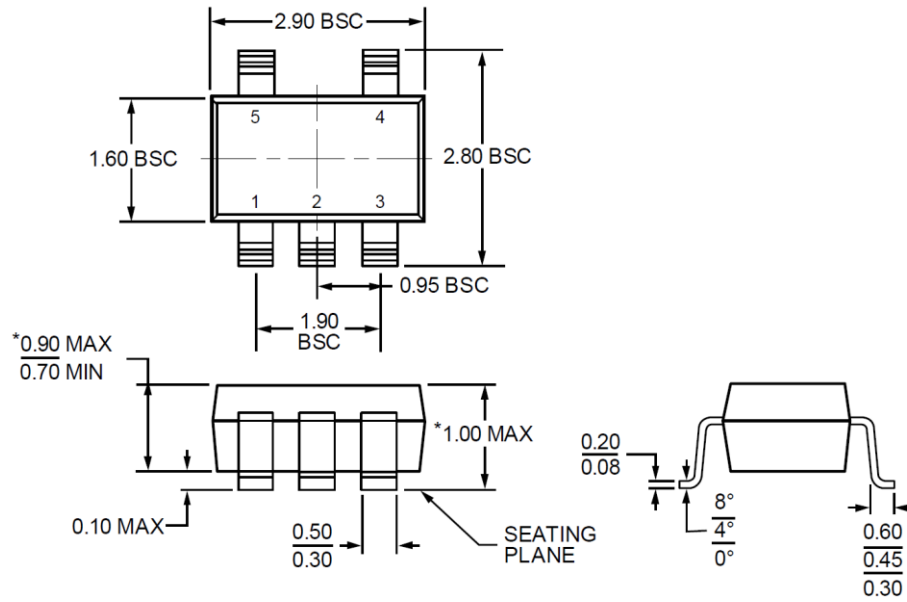
图 31.5 引脚超薄 SOT
