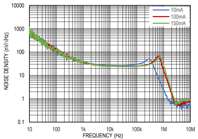
图 17. 输出噪声谱密度, V_{IN}=5\text{V} , V_{OUT}=3.3\text{V}
