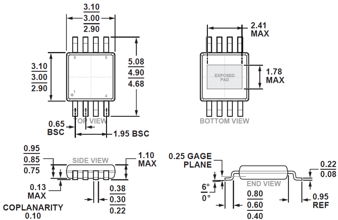
图 32.8 引脚 MSOP
