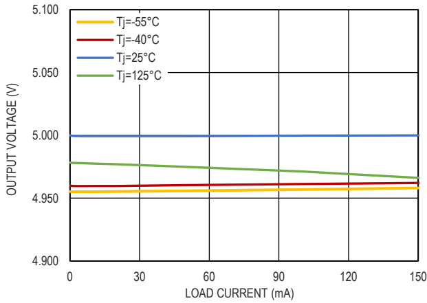
图 12. 5.0V 输出电压和负载电流的关系
