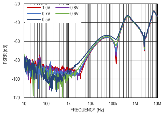
图 18. 电源电压纹波抑制比与压差的关系, V_{OUT}=3.3V
