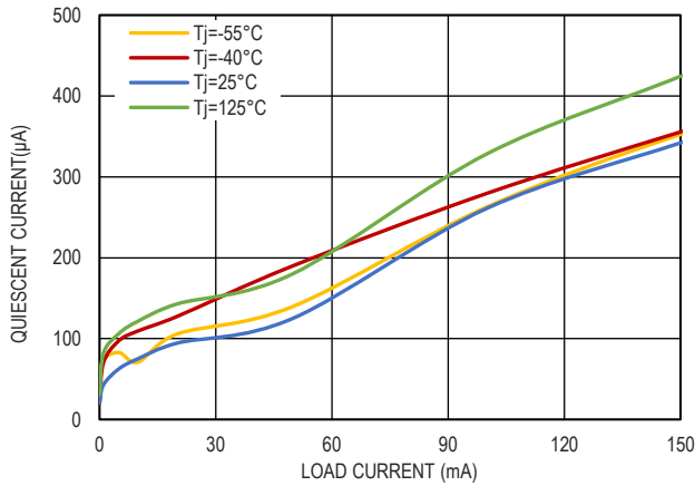
图 8. 静态电流和负载电流的关系, V_{IN} = 4.3V
