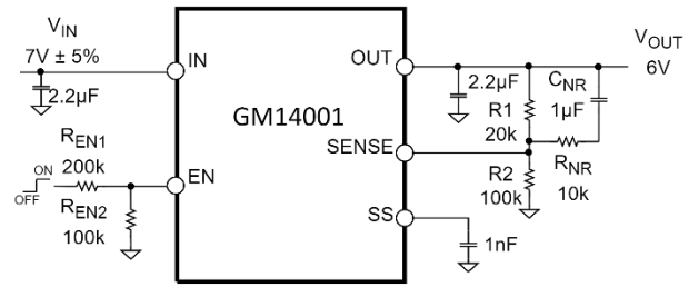
图 29. 噪声优化
