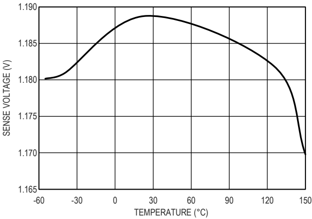
图 14. 1.188V SENSE 引脚电压精度
