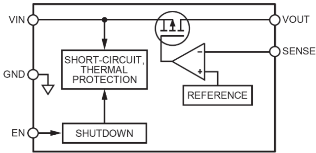
图 23. 内部框图
