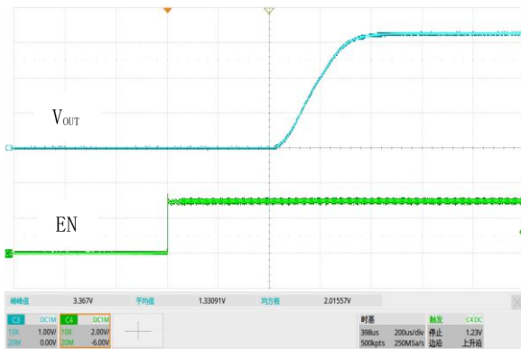
图 21. 软启动, V_{IN}=4.3V , V_{OUT}=3.3V , I_{OUT}=300mA
