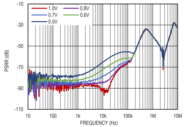
图 18. 电源电压纹波抑制比与压差的关系, V_{OUT}=5.0V
