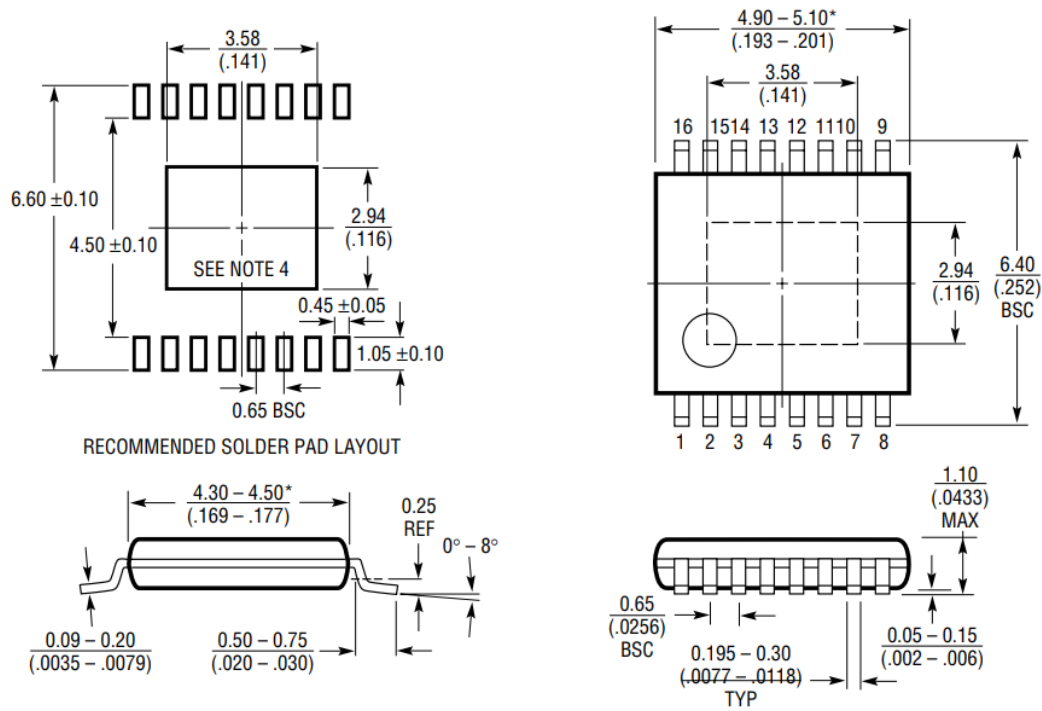
图 22. 16 引脚 TSSOP
