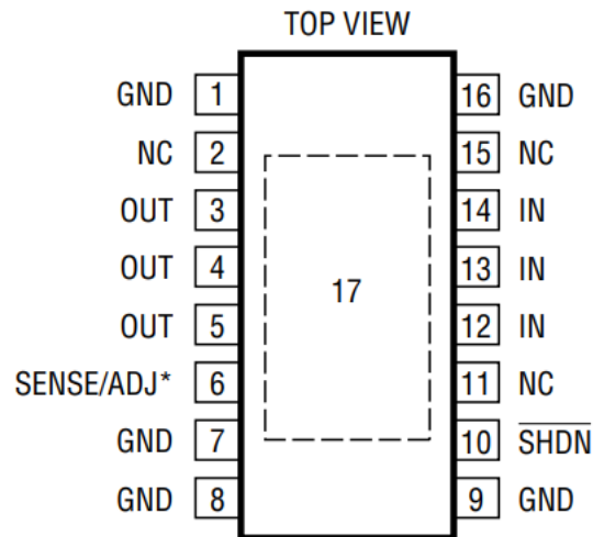
图 3 引脚配置
