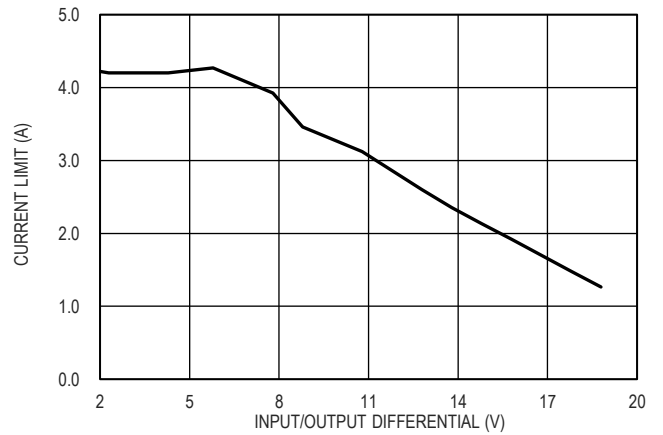
图 13. 输出限流值和输入输出压差的关系
