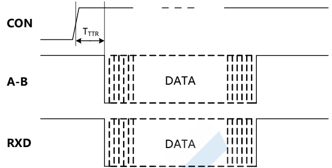
图 2. RSM(3)485EHT模块数据接收时序图
