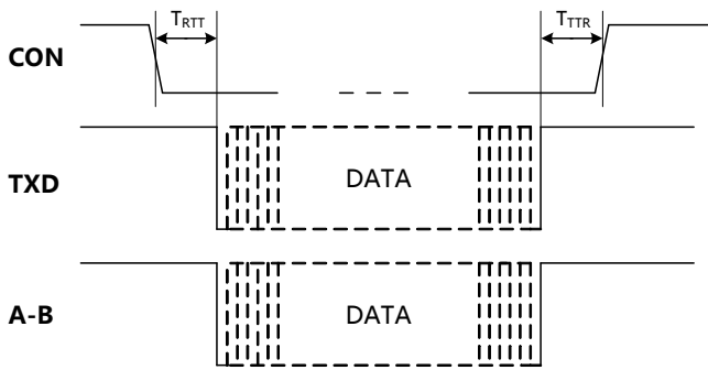
图 1. RSM(3)485EHT模块数据发送时序图
