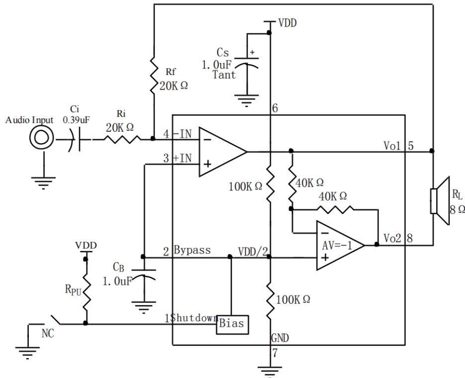
图 1、LM4861B 典型应用图
