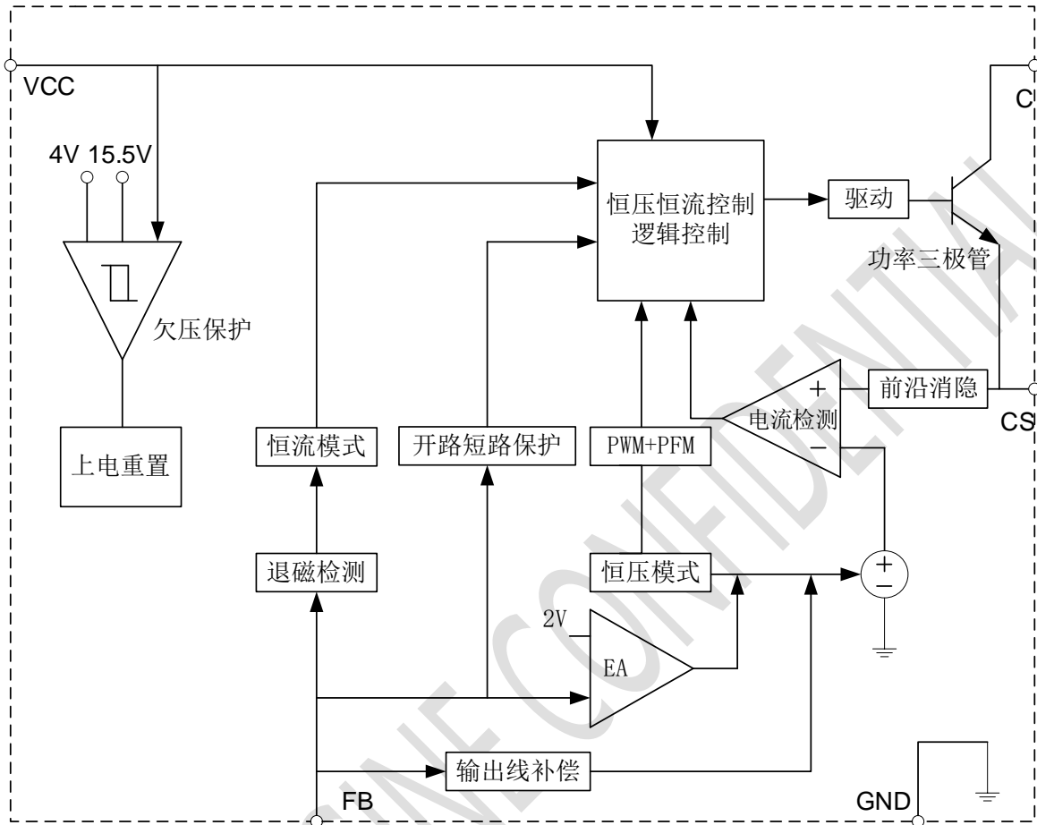
图3 SZ2525X 内部框图
