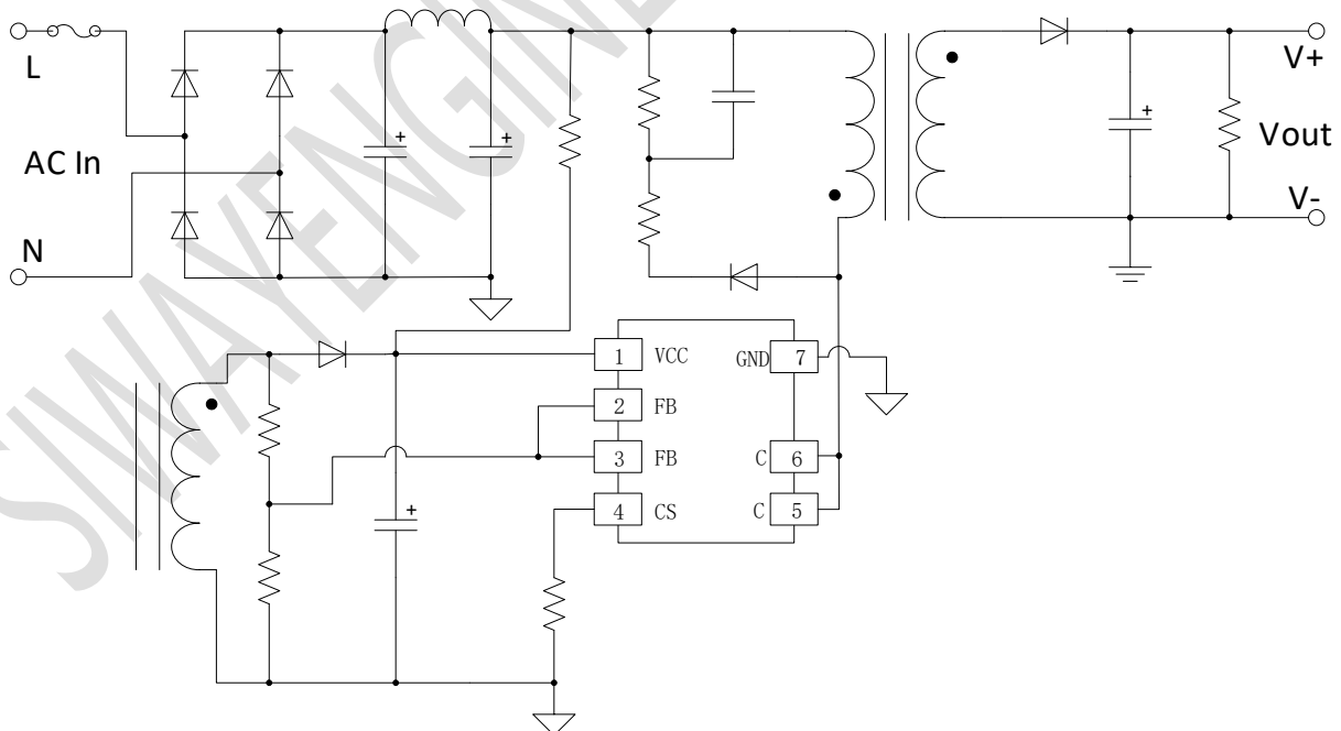
图 1 SZ2525X 典型应用图
