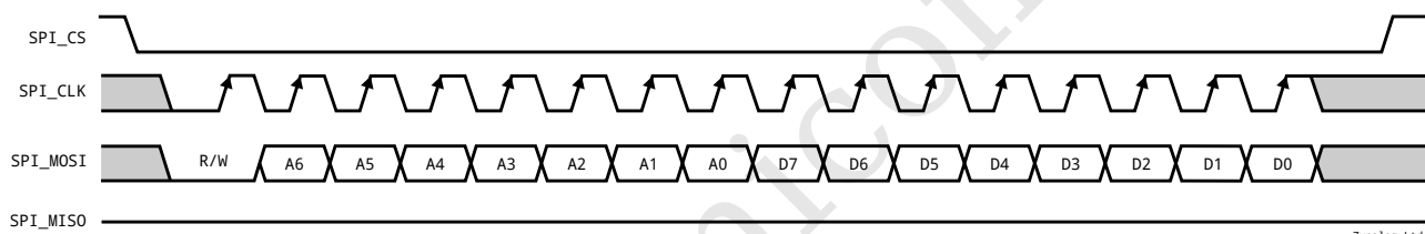
写入时序
