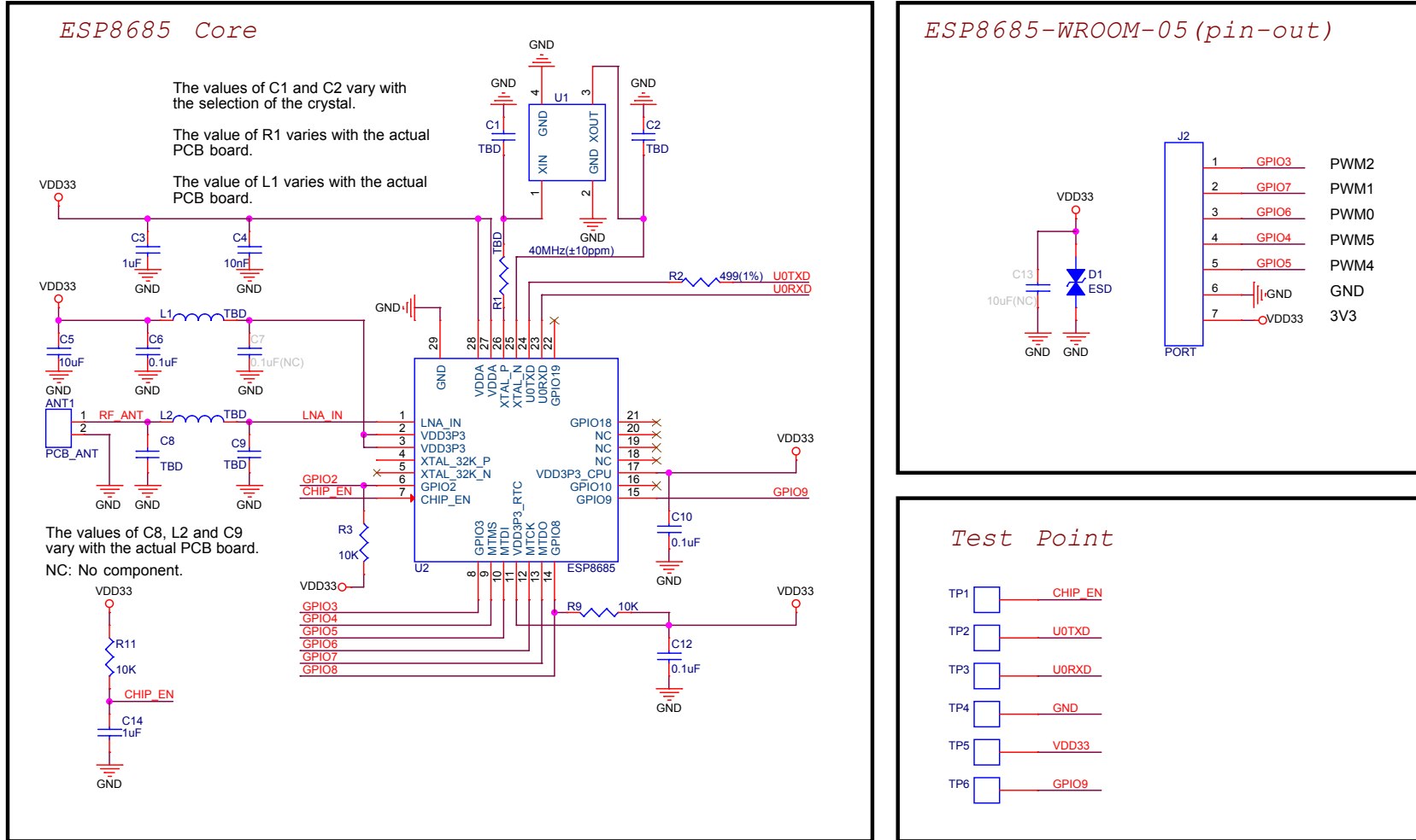
图 4: ESP8685-WROOM-05 原理图
