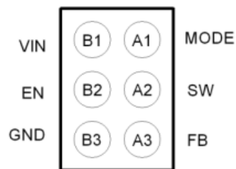
图 4. 底视图
