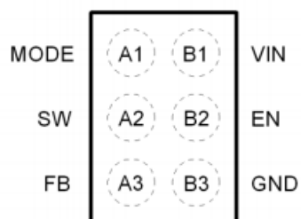
图 3. 顶视图
