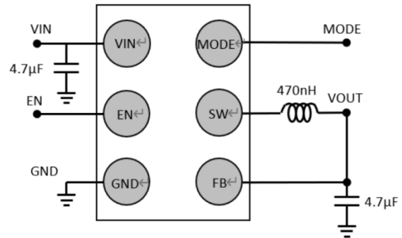
图1. 典型应用
