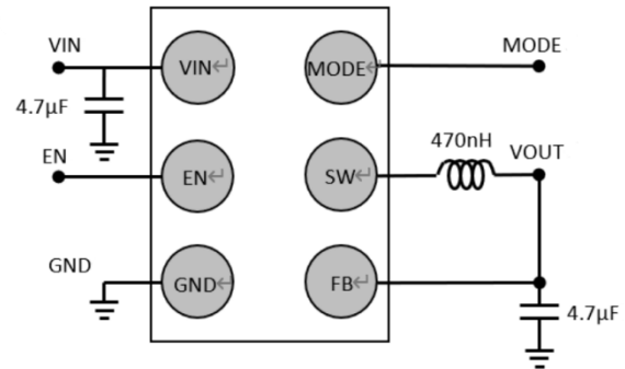
图1. 典型应用
