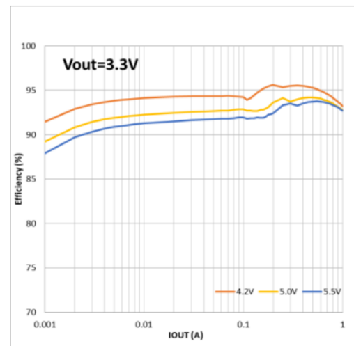
图2. 典型效率, Mode = Low
