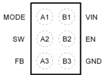
图 3. 顶视图
