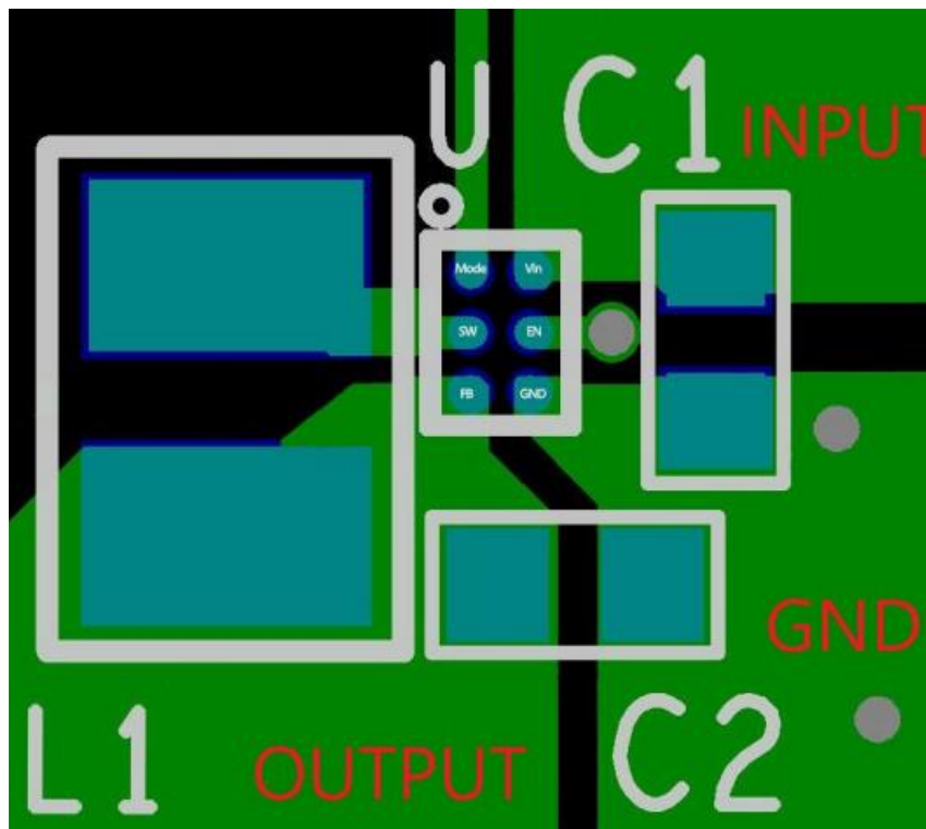
图 45. 顶层布局
