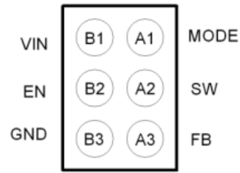
图 4. 底视图
