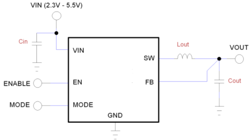
图 44. 应用电路
