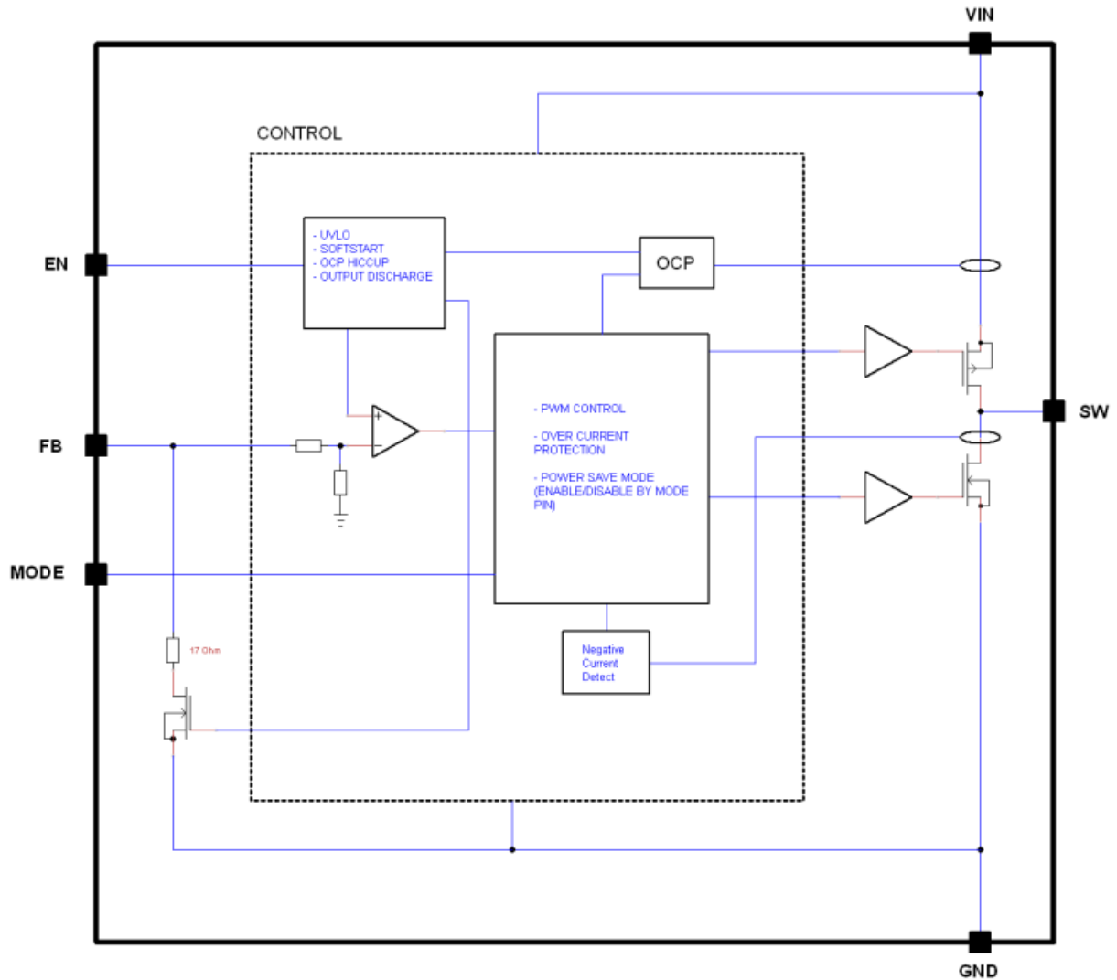
图 43. 功能框图
