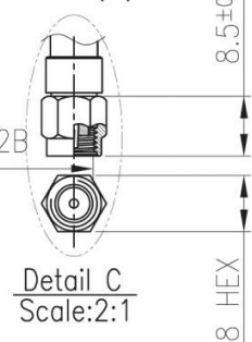
RP-SMA(M)ST
