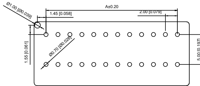
P.C.B LAYOUT
