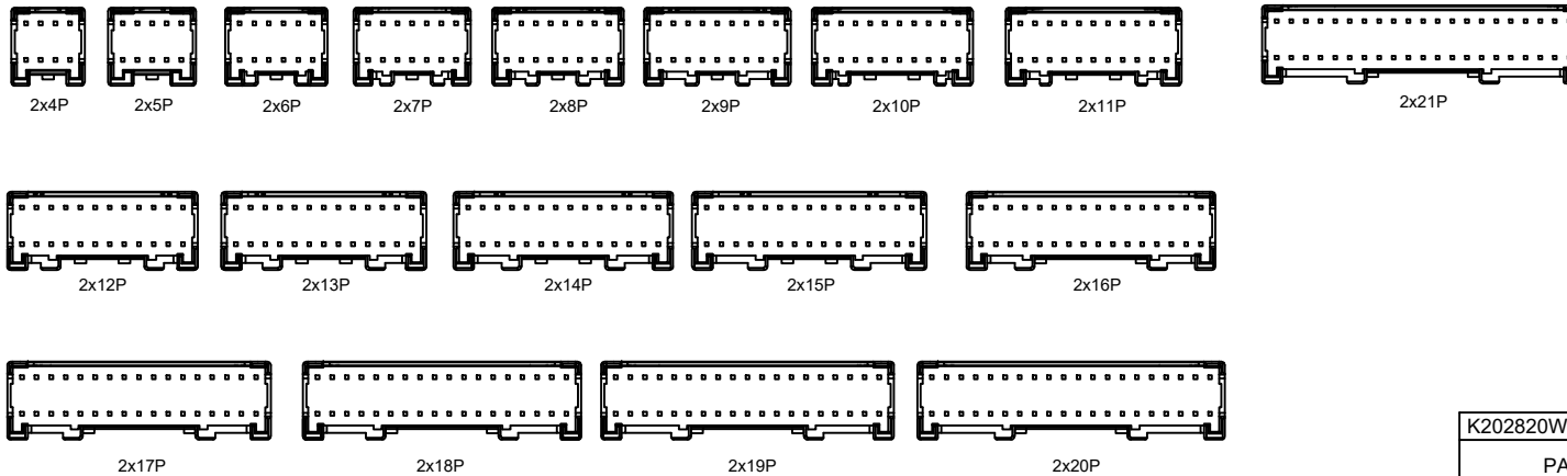
P.C.B LAYOUT
