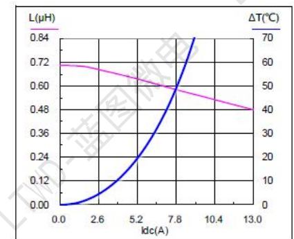
SMS0420-R68M
