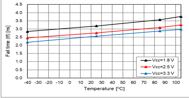
10% - 90% V CC , L CMOS = 15 pF, Temp. Char.
