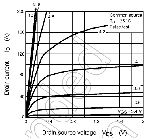
Fig. 9.2 I_D - V_{DS}
