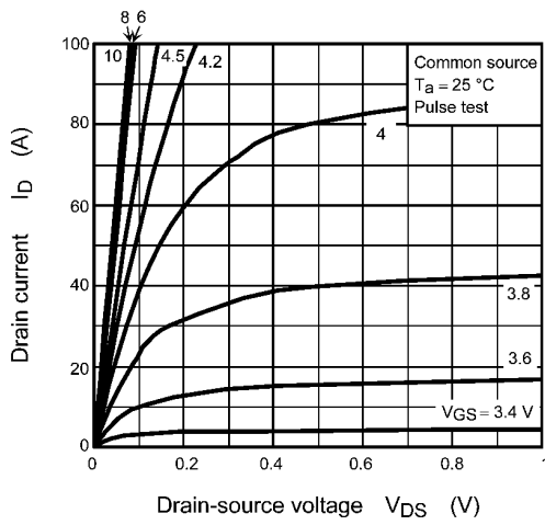
Fig. 9.1 I_D - V_{DS}
