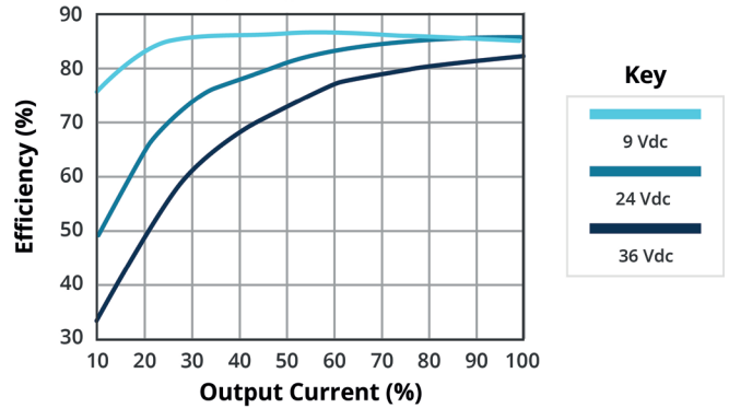
EFFICIENCY VS OUTPUT LOAD PDQ10-Q24-S12-D
