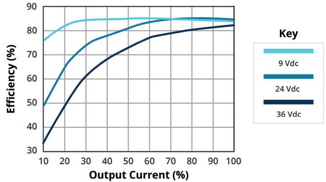
EFFICIENCY VS OUTPUT LOAD PDQ10-Q24-D5-D
