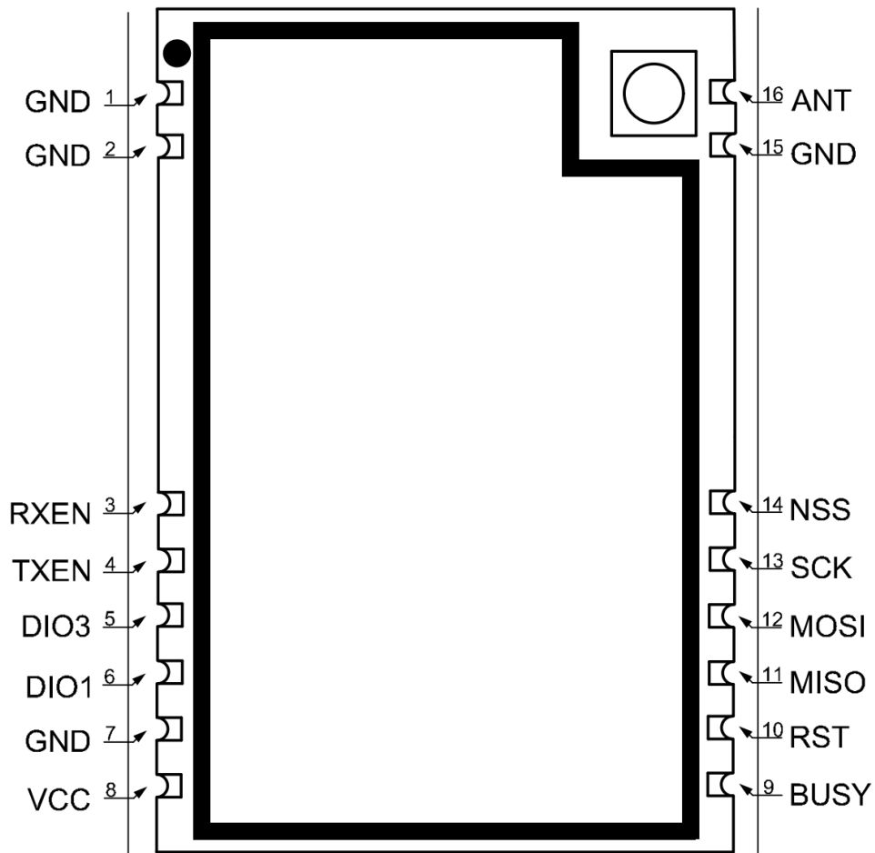
图 1-1 俯视图
