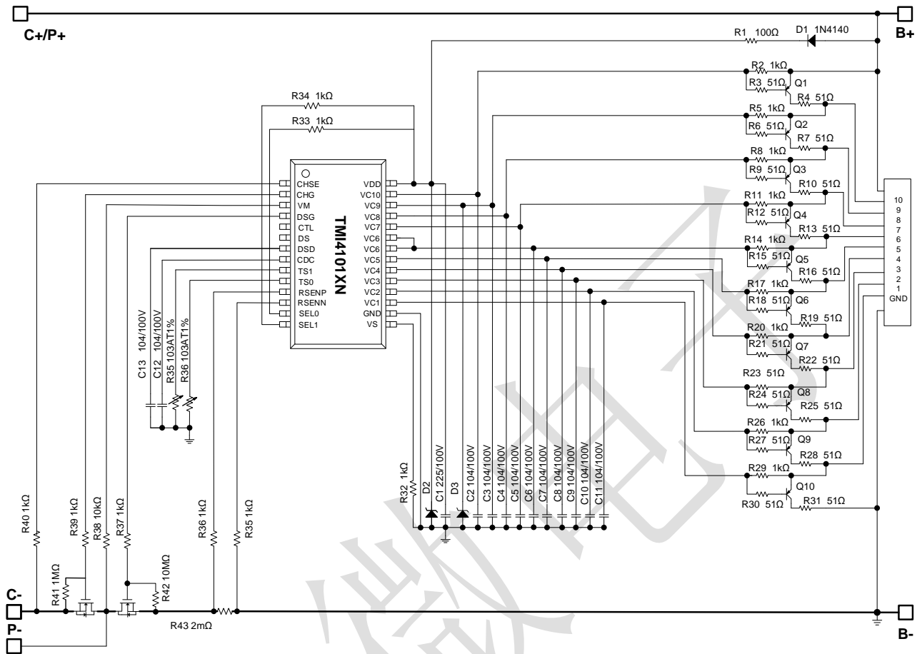
图5 TMI4101XN典型应用图(10串分口)
