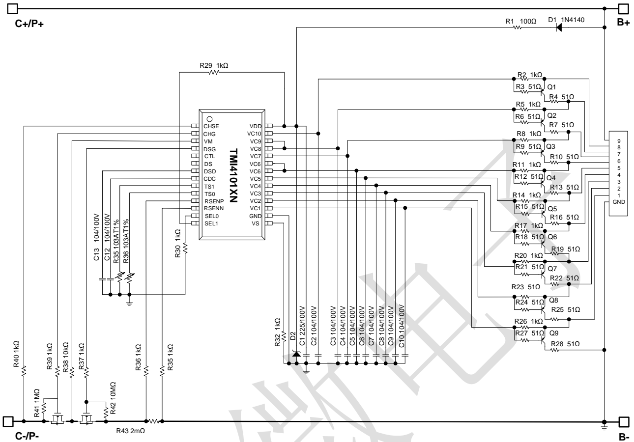
图2 TMI4101XN典型应用图(9串同口)
