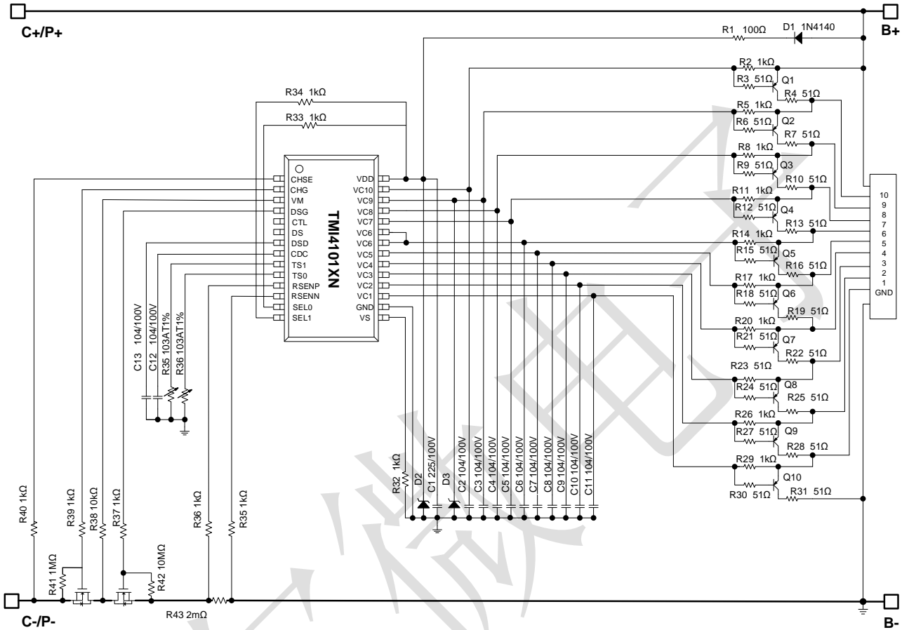
图1 TMI4101XN典型应用图(10串同口)
