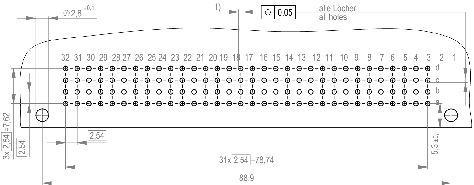
Leiterplatten-Lochbild / PCB drillhole pattern
