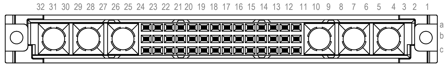
Bestückungsplan / contact layout
