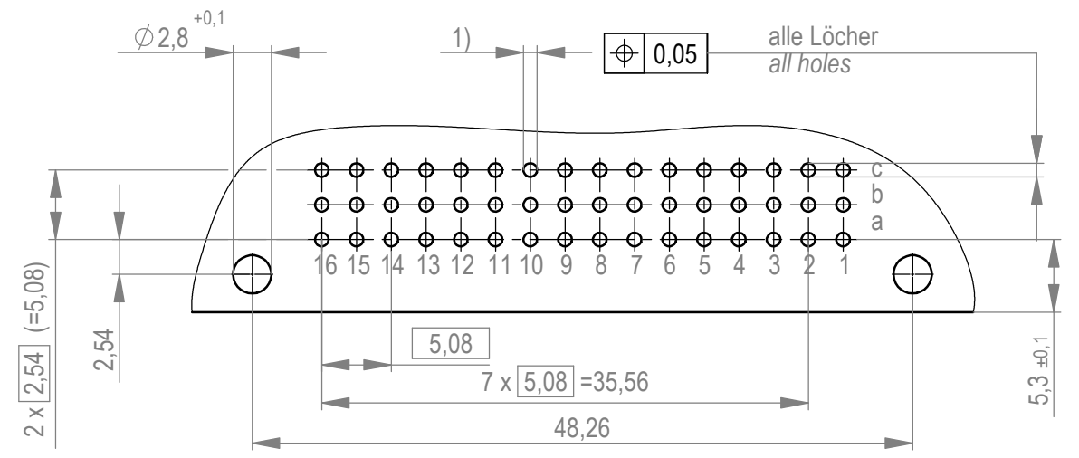
Leiterplatten- Lochbild / PCB drillhole pattern
