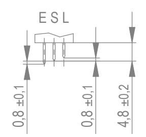
Stecklänge / mating length
