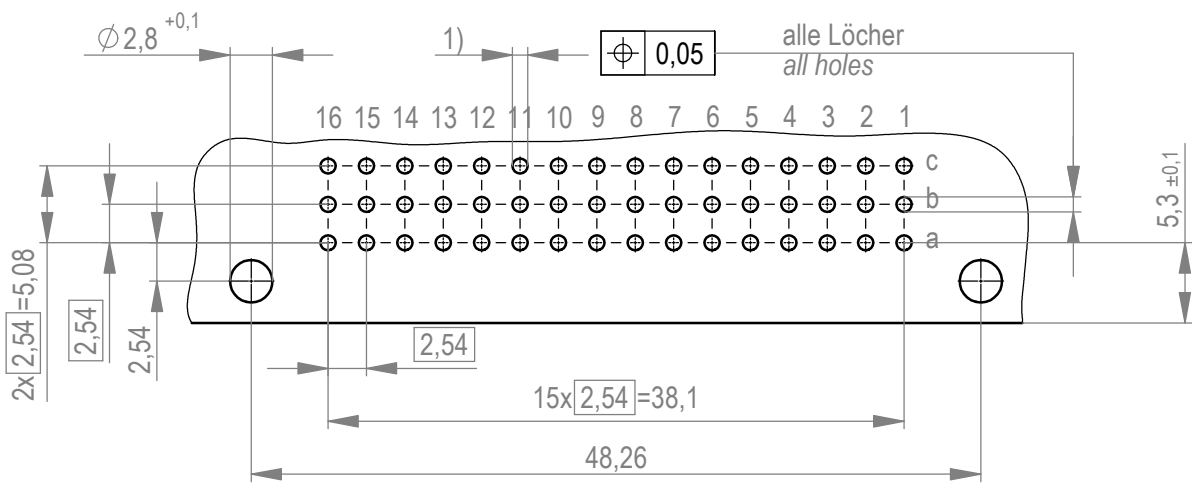
Leiterplatten-Lochbild / PCB drillhole pattern
