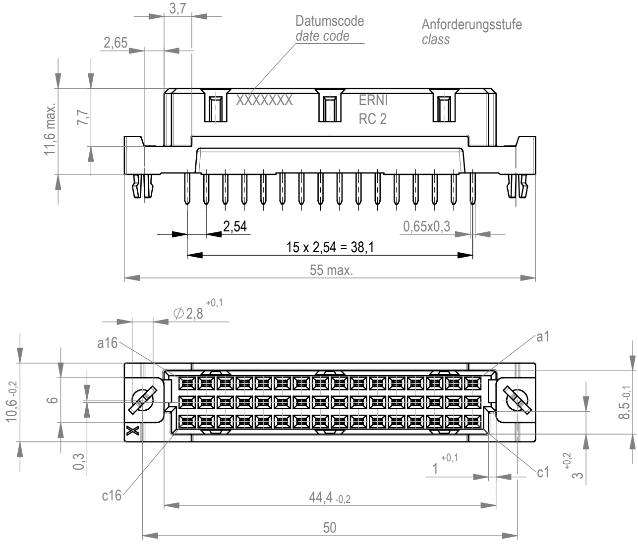
Bestückungsplan / contact layout
