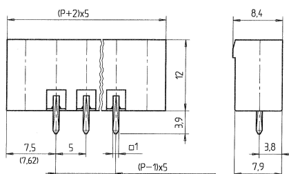
P=Polzahl/poles/plots
