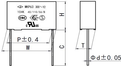
W±0.4, H±0.4, T±0.4 方底(Square-bottom)
