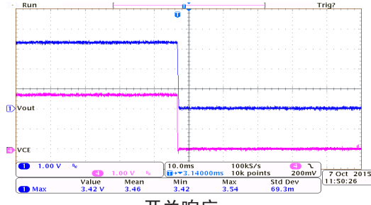
开关响应: HT7533-7 ( I_{OUT}=100mA , V_{CE}=2.7V to 0V)
