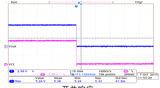
开关响应: HT7550-7 ( I_{OUT}=150mA , V_{CE}=2.7V to 0V)
