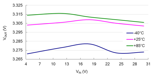
电压线性调整率: HT7333-2 ( I_{OUT}=10mA )
