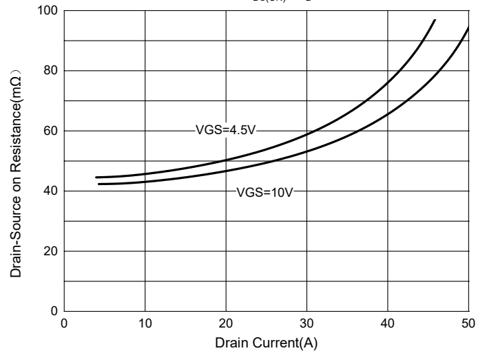
Fig. 4 - R_{DS(ON)} - I_D
