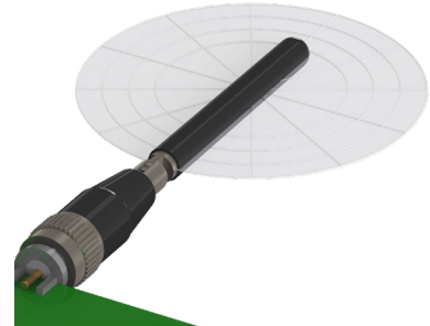
XZ-Plane Gain
