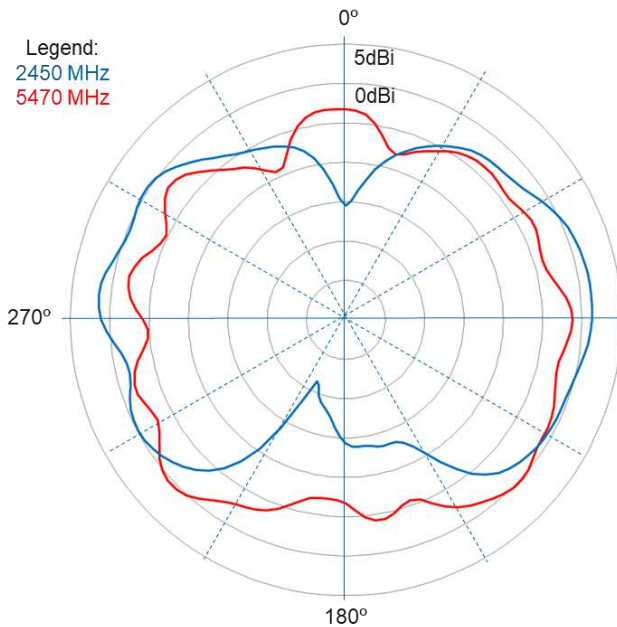
Elevation 1
