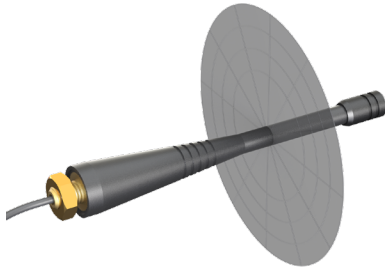
XZ-Plane Gain
