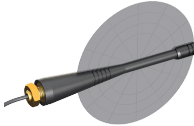
YZ-Plane Gain
