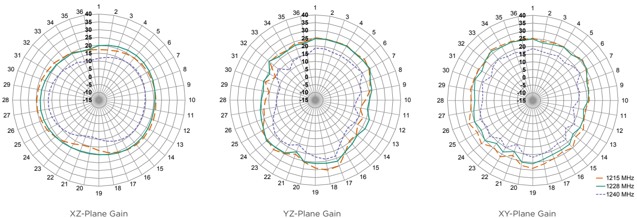
XZ-Plane Gain
