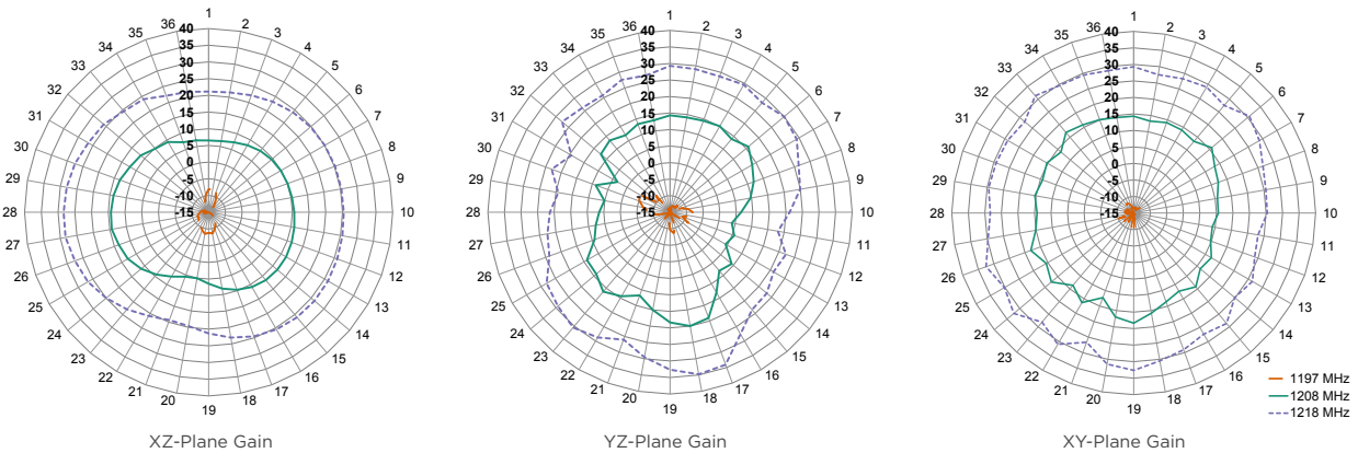
XZ-Plane Gain
