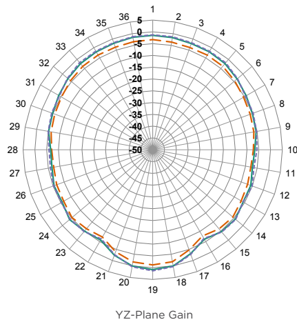
YZ-Plane Gain
