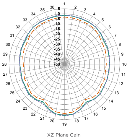
XZ-Plane Gain
