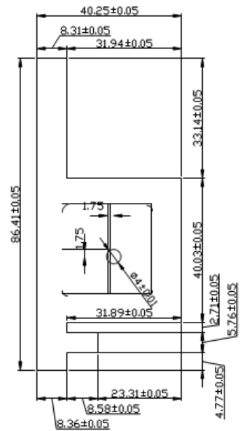
Top side
