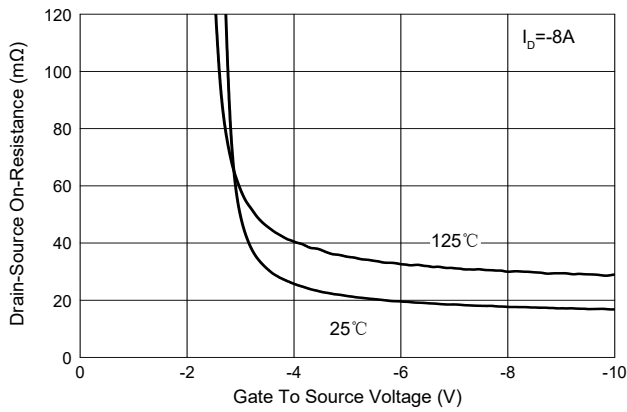
Fig.3 - R_{DS(ON)} - V_{GS}
