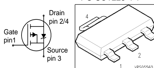
PG-SOT223-4-1
