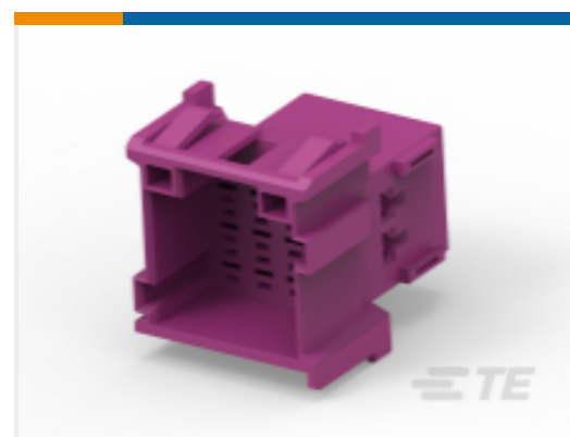
TE Part #1-967627-6 FLACHSTE-GEH2,8 12P
