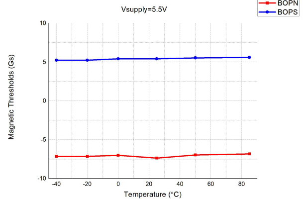
磁场阈值 vs 温度 @VDD=5.5V
