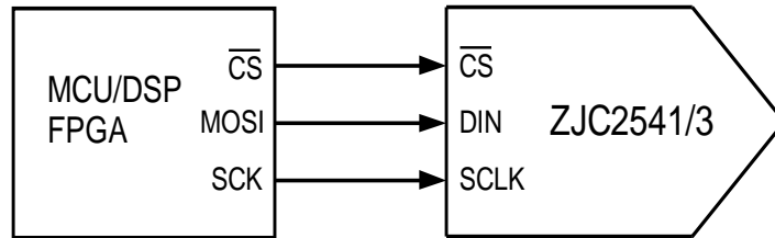
图37. ZJC2541/3 与控制器接口的连接
