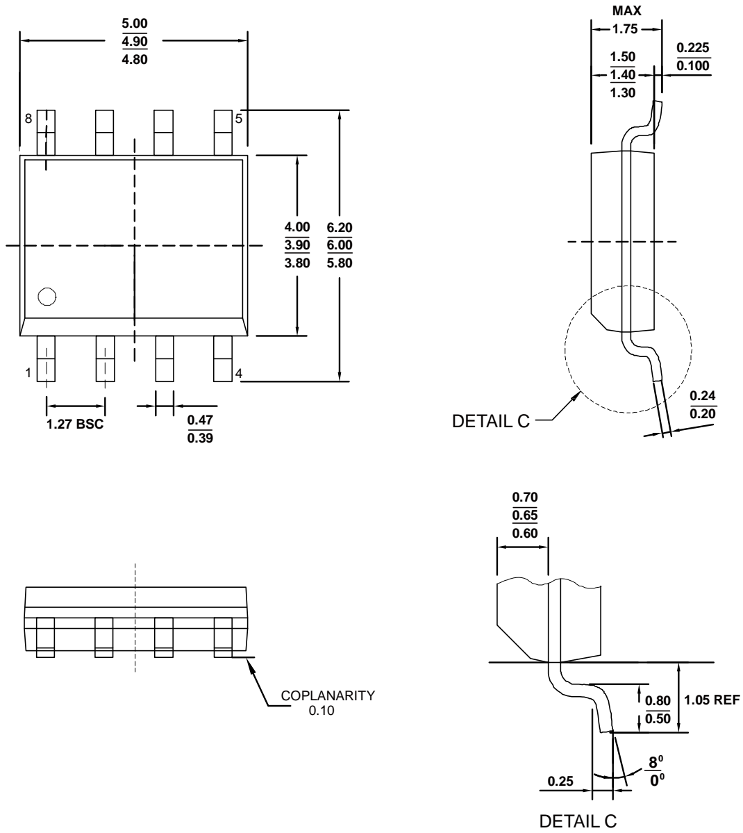
图38. SOIC-8 封装尺寸图 (单位: 毫米)
