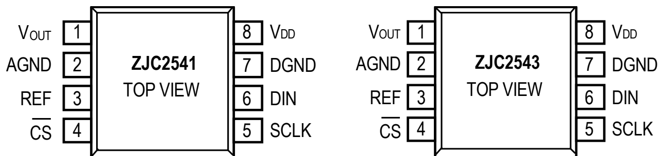
图3. ZJC2541 和 ZJC2543 具有相同的 8 引脚 SOIC 管脚配置图
