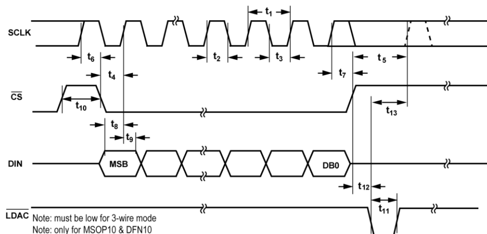
图6. 数字接口时序
