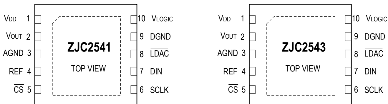
图5. ZJC2541 和 ZJC2543 具有相同的 10 引脚 DFN 管脚配置图
