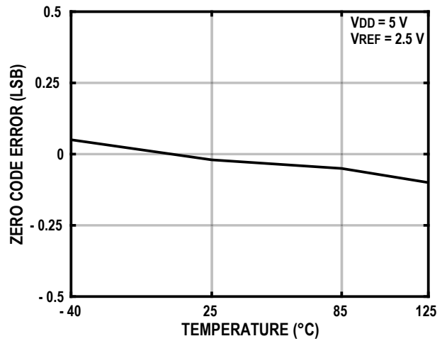
图18. 零代码误差与温度的关系-16位
