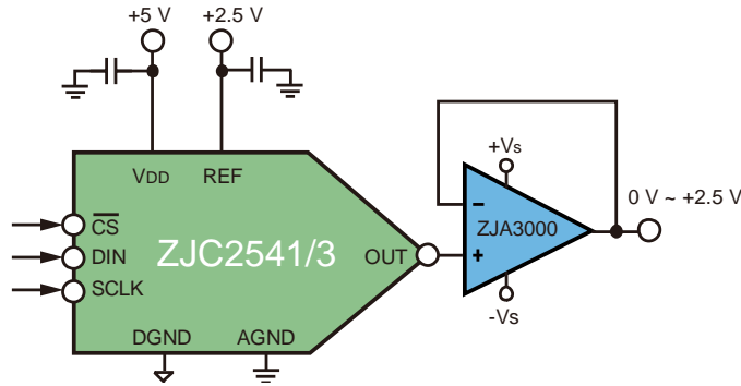
图36. 典型输出连接
