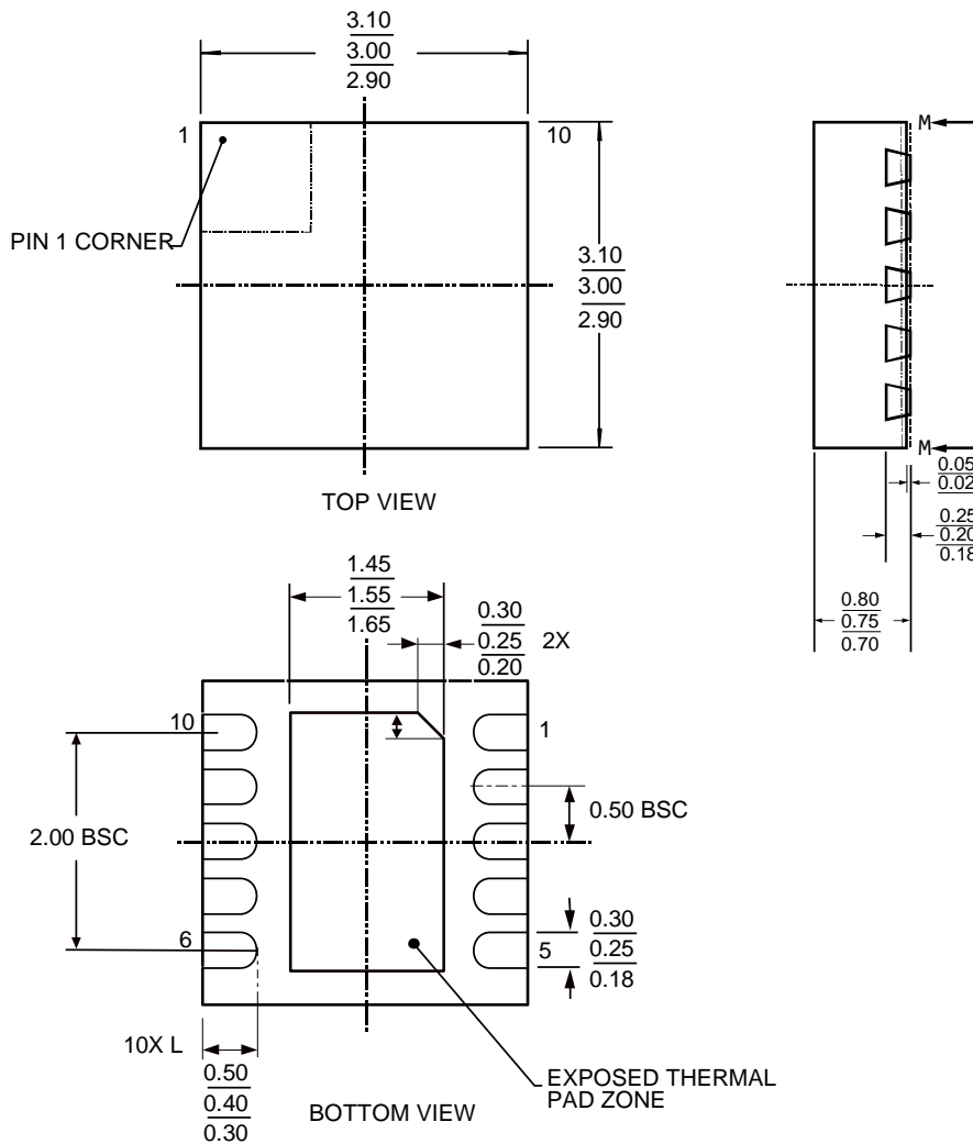
图40. DFN-10 封装尺寸图 (单位: 毫米)
