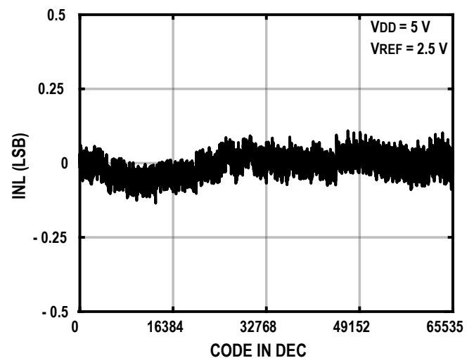
图2. ZJC2541/3-16 INL
