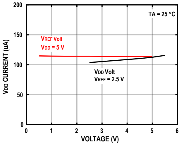
图25. 电流与电源电压的关系
