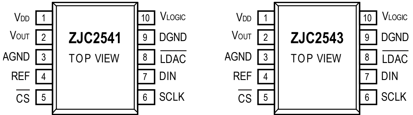
图4. ZJC2541 和 ZJC2543 具有相同的 10 引脚 MSOP 管脚配置图
