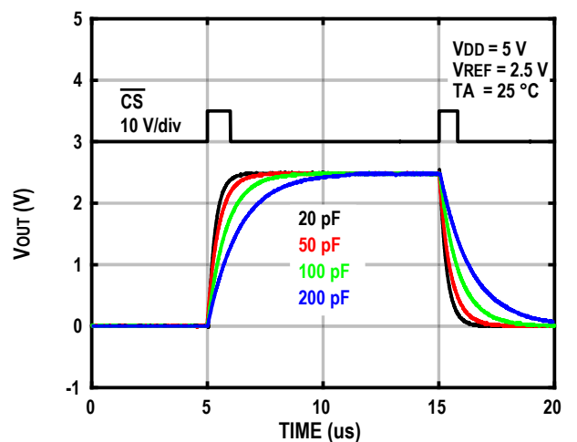
图30. 大信号建立时间
