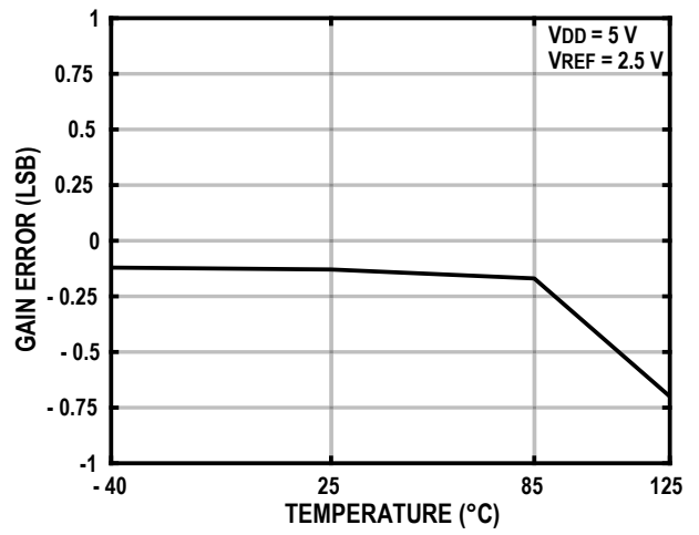
图16. 增益误差与温度的关系-16位
