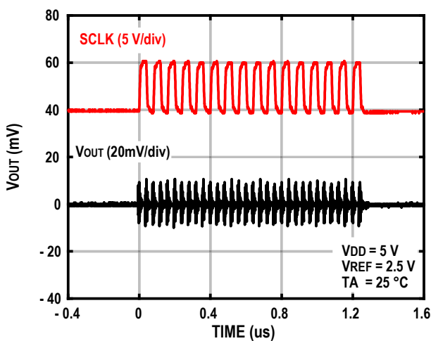
图29. 数字反馈
