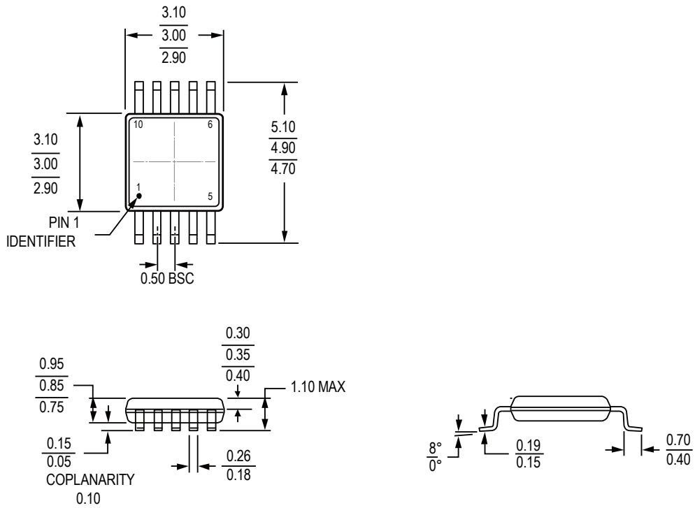
图39. MSOP-10 封装尺寸图 (单位: 毫米)
